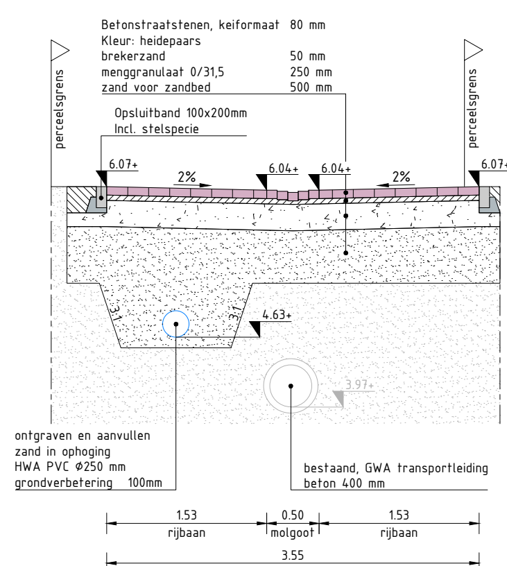
Dwarsprofiel A-A
