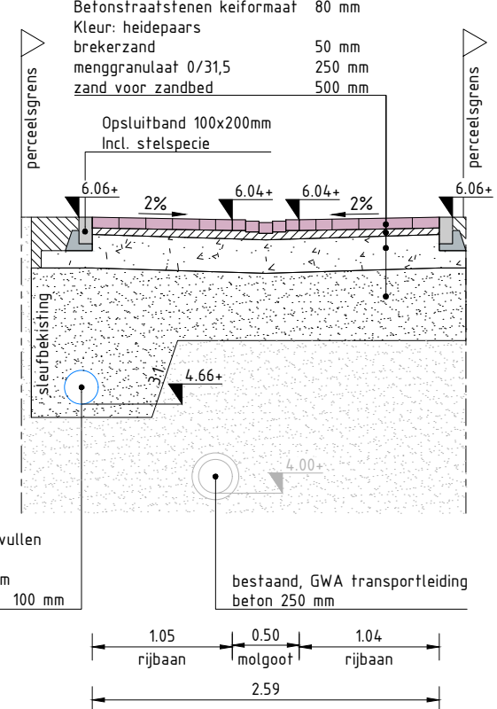
Dwarsprofiel B-B
