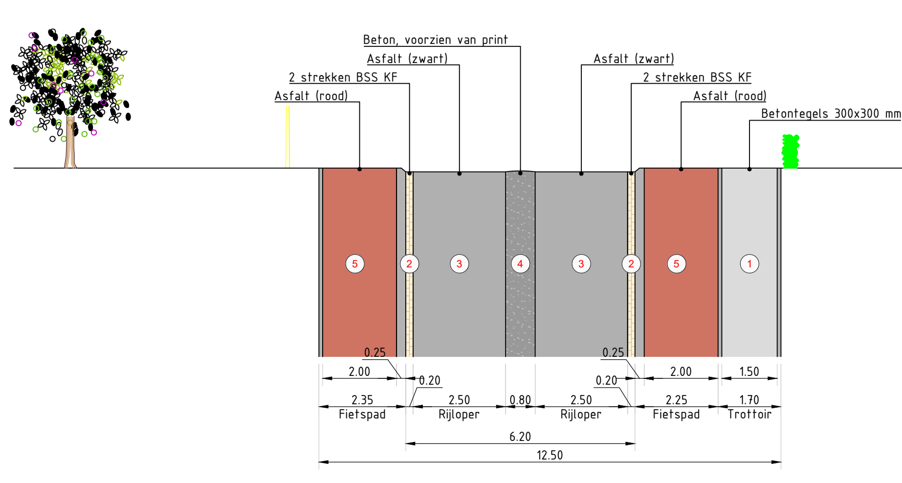
Principeprofiel C-C (Vogelenzangseweg Zuid) Schaal 1:100
