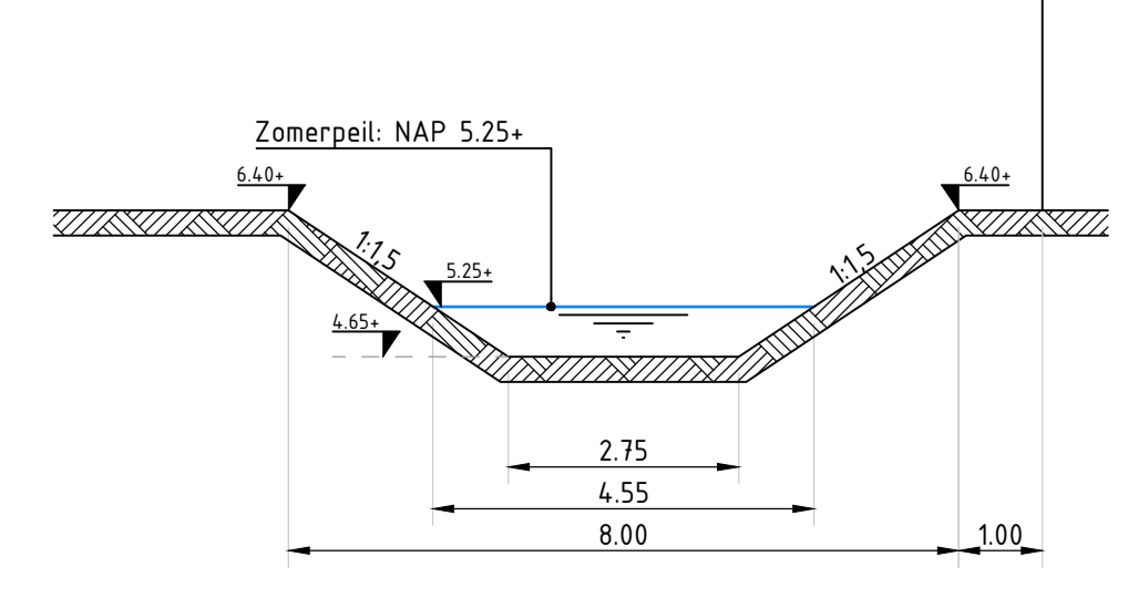
Principeprofiel D-D Schaal 1:100
